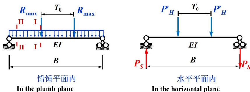
图 4.1 端梁的计算简图
