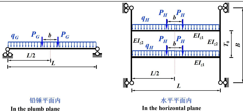
图 3.2 主梁的计算简图
