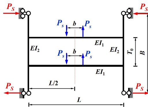
图 2.2 大车偏斜运行时的水平侧向力作用图
