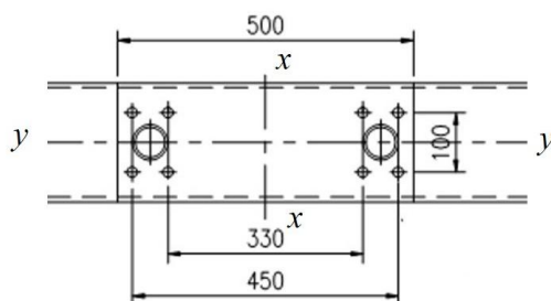
图 5.1 螺栓群的布置图
